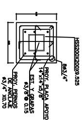
DETALLE DE PEDESTAL
