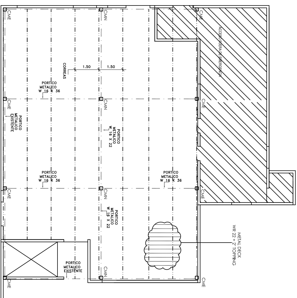
DETALLE DE METALDECK
